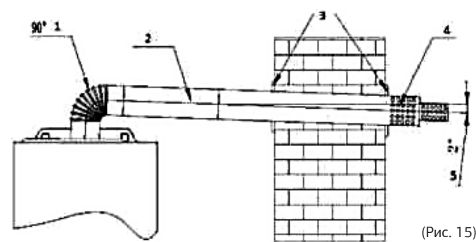
1 - 90° патрубок; 2 - Удлинение трубы дымоотвода; 3 - фланцы трубы дымоотвода; 4 - труба дымоотвода; 5 - Уклон вниз 2°.
