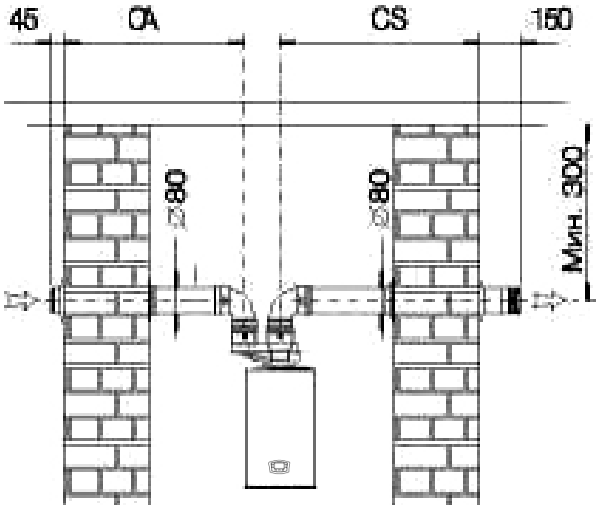
Воздухозабор и дымоотвод через стену
