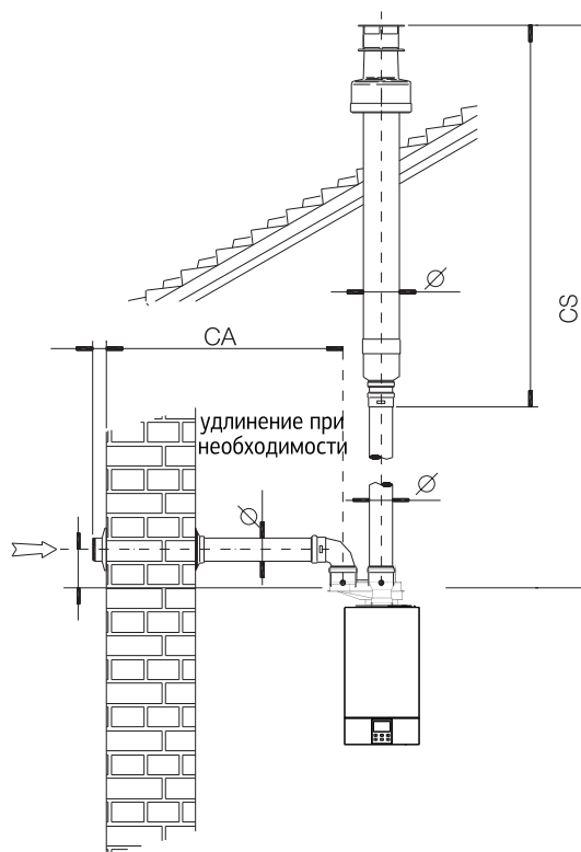
Раздельная система воздухозабора и вертикальным дымоходом
